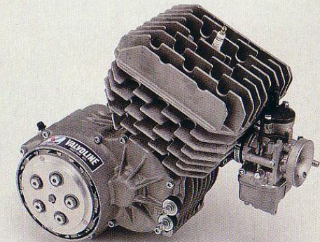
MOTORE KART 125 CATEGORIA NAZIONALE
