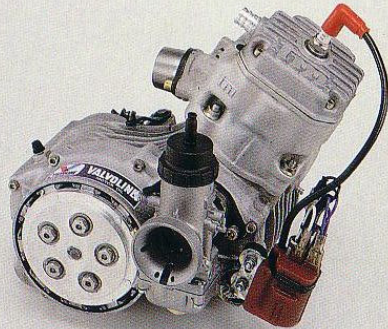
MOTORE KART 125 C-1-C INTERNAZIONALE
