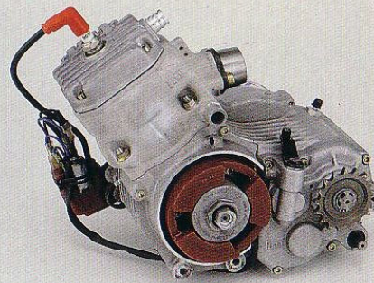
MOTORE KART 125 C-1-C INTERNAZIONALE
